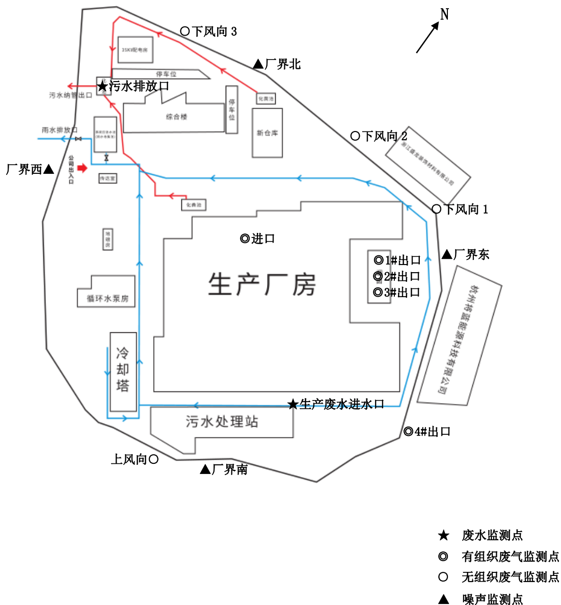
图 7-3 监测点位布置图
