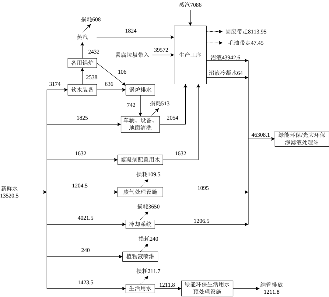
图 3-5 项目水平衡图
