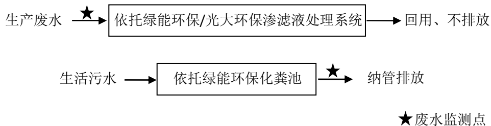
图 7-1 废水监测点位布置图
