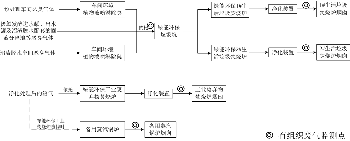
图 7-2 废气监测点位布置图
