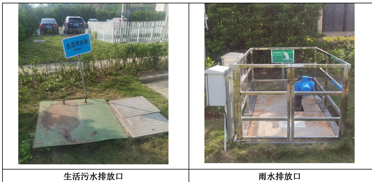
图4-2 生活污水排放口、雨水排放口照片
