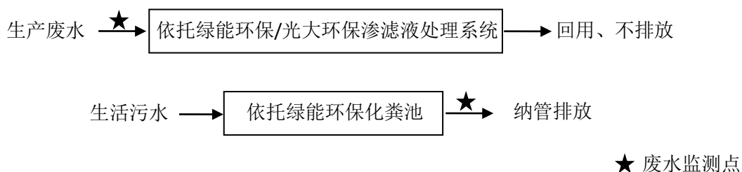
图4-1 实际污水处理工艺流程图
