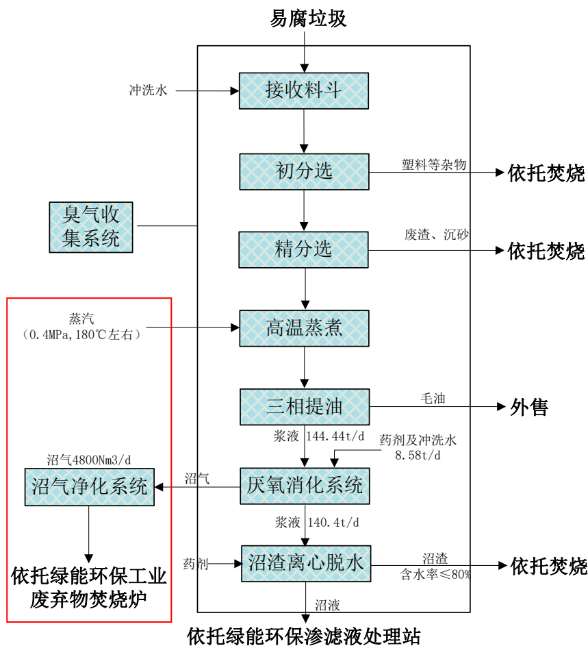
图 3-4 项目工艺流程图
