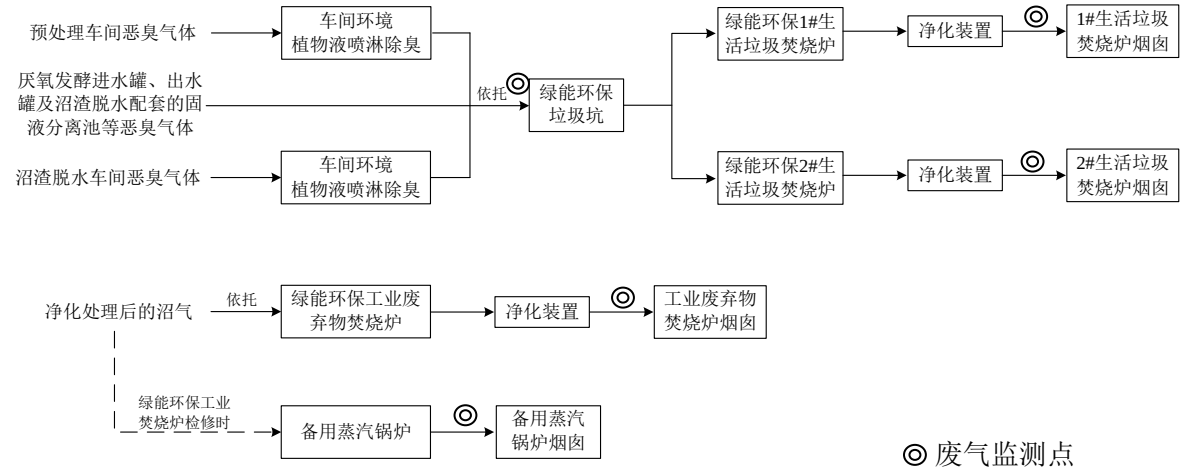
图4-3 项目废气处理及排放流程图
