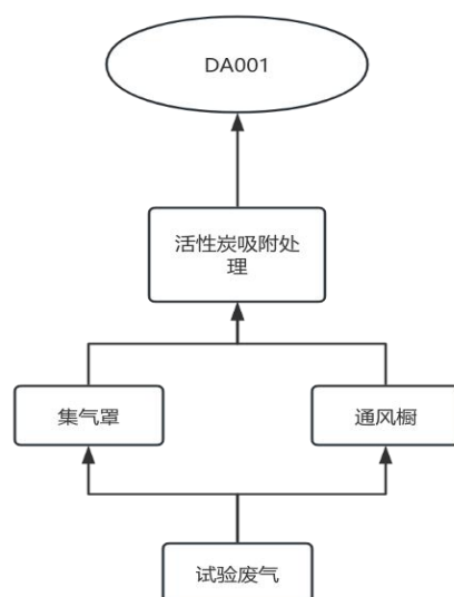
图 4-1 废气治理设施
