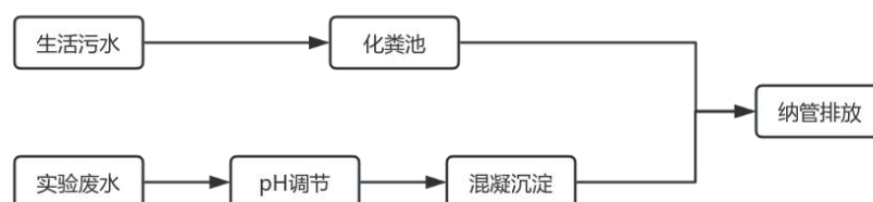
图 4-2 项目废水处理工艺流程图
