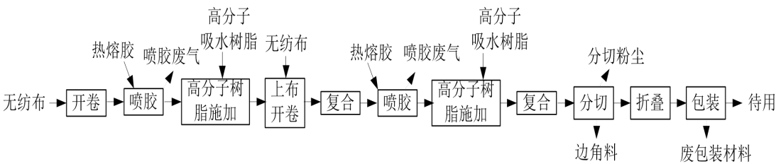
图 2-9 现有项目复合芯体生产工艺流程
