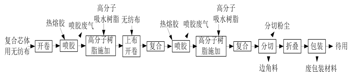
图 2-2 项目复合芯体生产工艺流程
