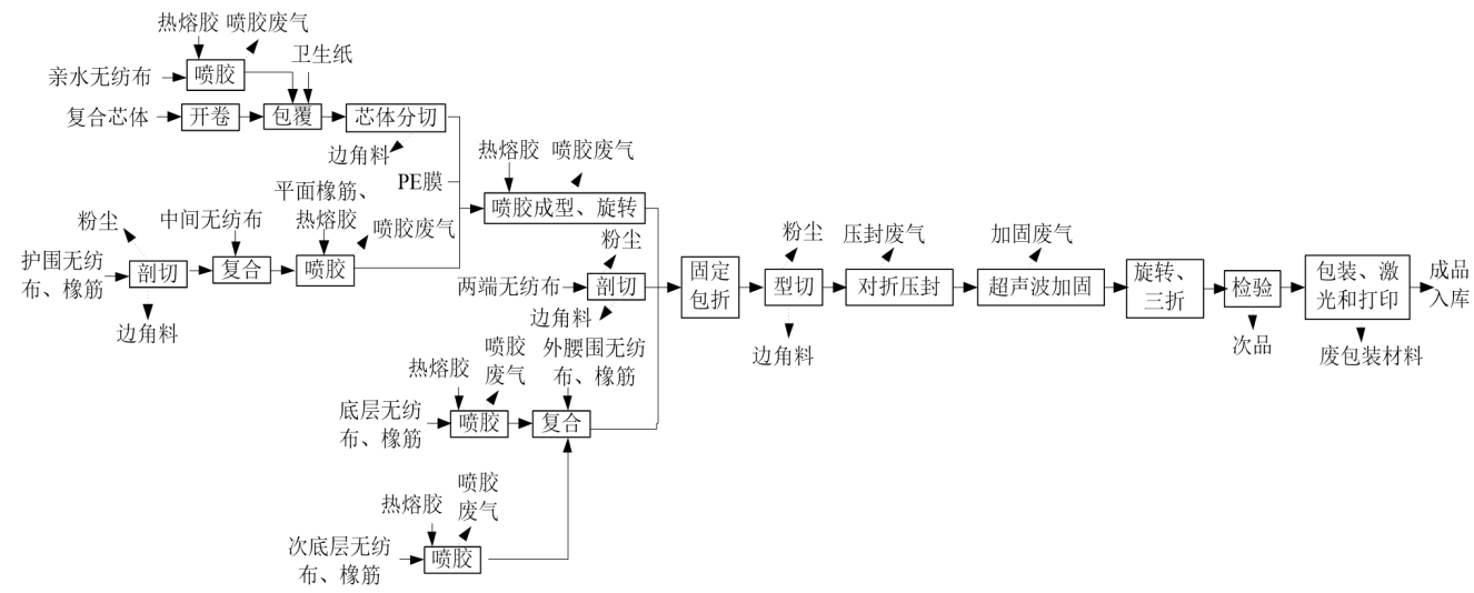
图 2-4 项目经期裤生产工艺流程
