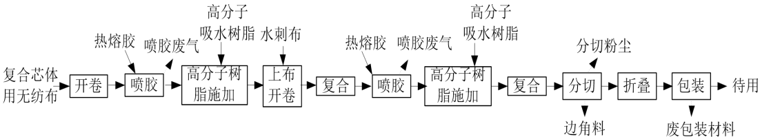
图 2-6 二厂复合芯体生产工艺流程
