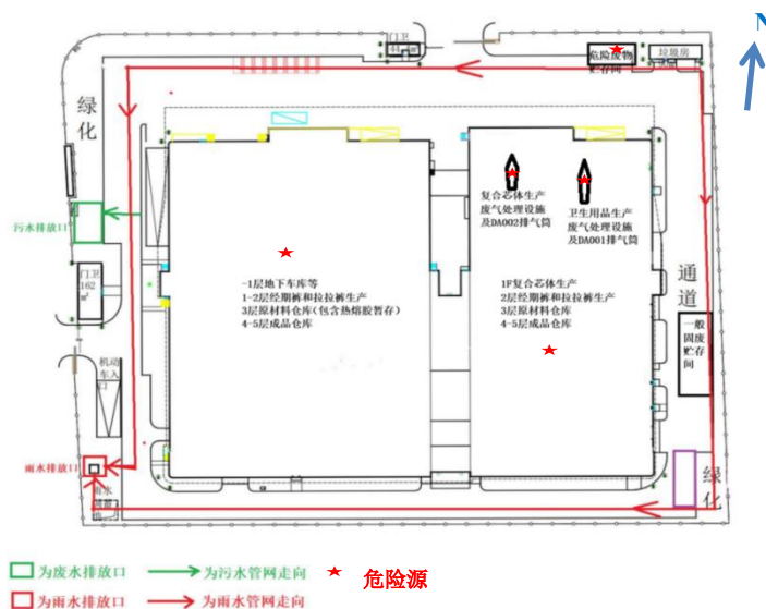
图 4-2 危险单元面分布图
