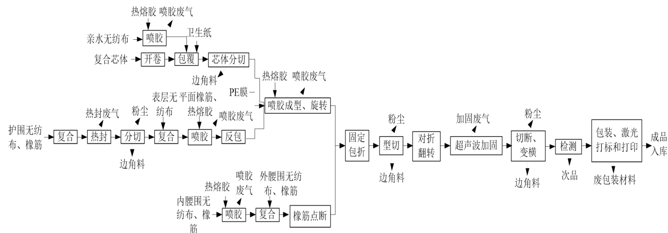
图 2-3 项目婴儿拉拉裤生产工艺流程
