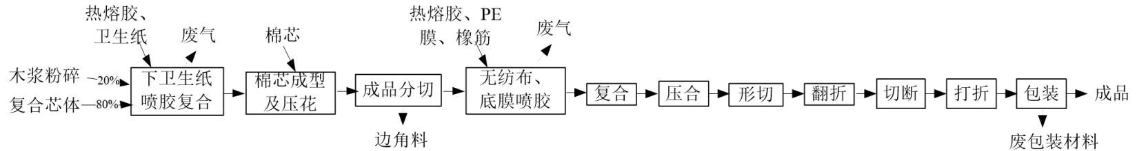
图 2-8 二厂裤型卫生巾生产工艺流程
