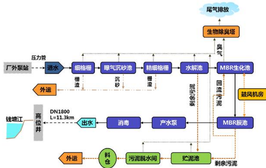
图 4-1 临平净水厂处理工艺流程
