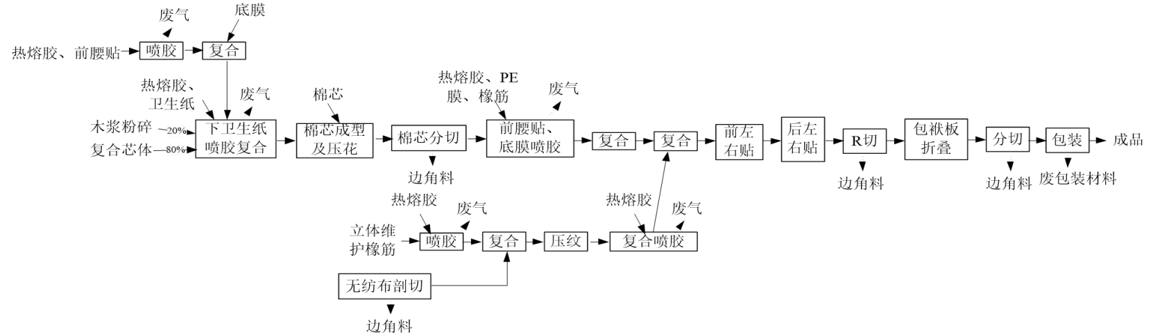
图 2-7 二厂拉拉裤生产工艺流程
